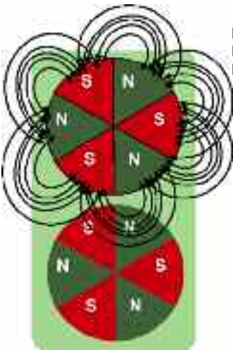
Magnetfeld mit radialverlaufender Polanordnung wechselnder Polarität
