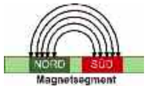
MAGNOFLEX® Magnetflußinduktion
